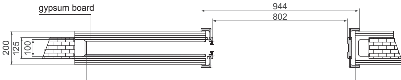
DOOR FRAME RANGE (126-200) – SYMMETRIC*
