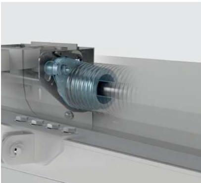
Zintegrowane zabezpieczenie przed pęknięciem sprężyn
