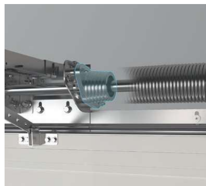
Zintegrowane zabezpieczenie przed pęknięciem sprężyn
