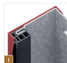
1 Boczna uszczelka + maskownica ościeżnicy w kolorze bramy
