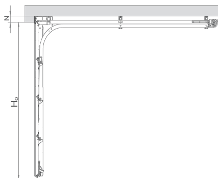
Montaż za otworem - maskownica za otworem
