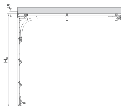
Montaż w otworze - maskownica przed otworem
