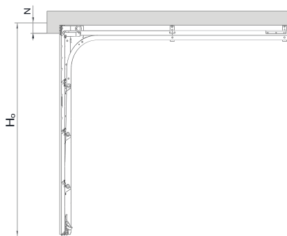
Montaż za otworem - maskownica za otworem
