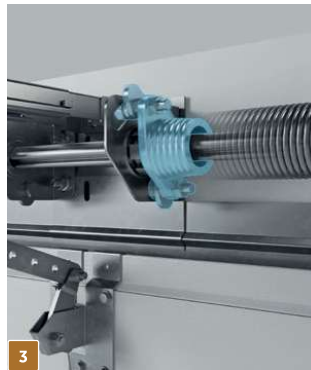
Zintegrowane zabezpieczenie przed pęknięciem sprężyn
