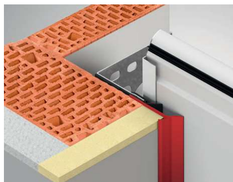
Uszczelnienie termiczne-wykańczające - opcja
