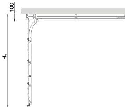
Montaż w otworze - maskownica w otworze
