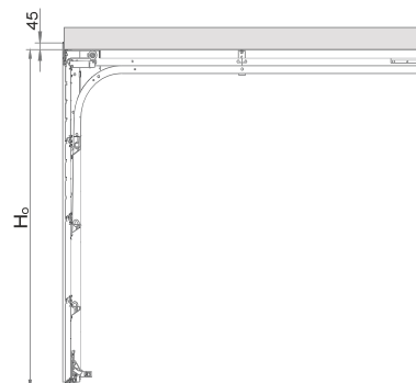
Montaż w otworze - maskownica przed otworem
