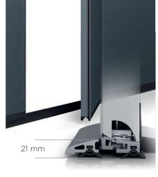
Niski próg w drzwiach przejściowych (o wysokości 21 mm)
